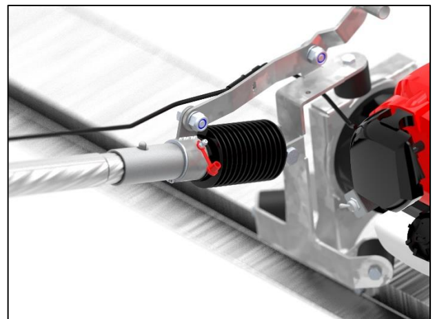
Detail beeld hoekverstelmechanisme
